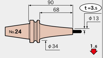
BT30-SLRA6-90 CV
